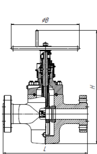
Без редуктора
