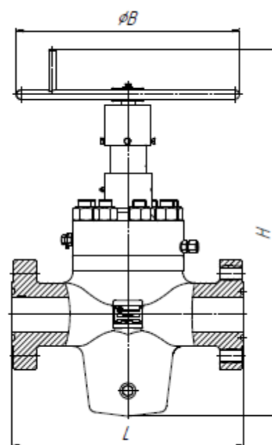
С редуктором
