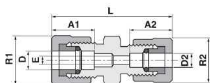
Переходное соединение
