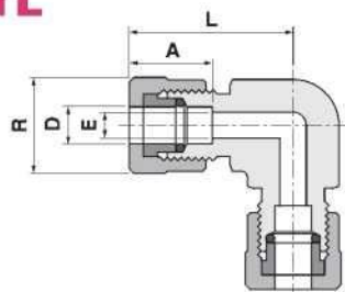
Коленчатое соединение
